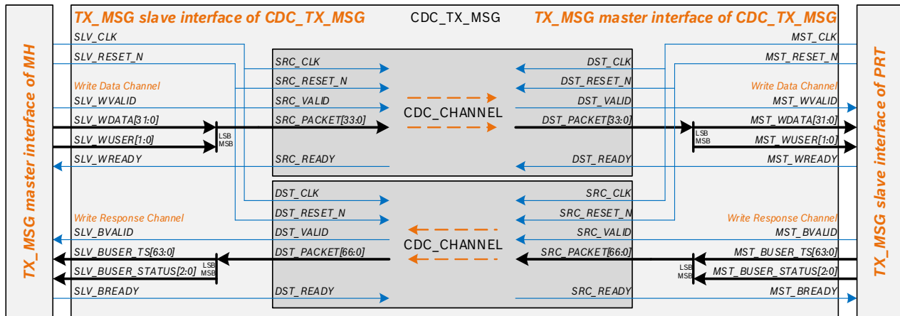
Figure 70. CDC_TX_MSG
